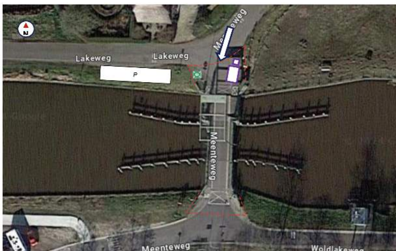
Figuur 3-1. Bouwplaatsinrichting Meenthebrug
